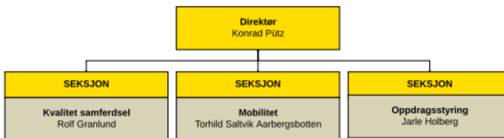
Figur 1. Organisasjonskart samferdselsavdelingen
